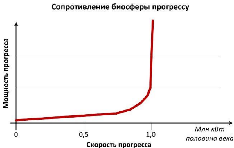
Рисунок 8. Сопротивление биосферы и геосферы Земли освоению новых уровней энергии
