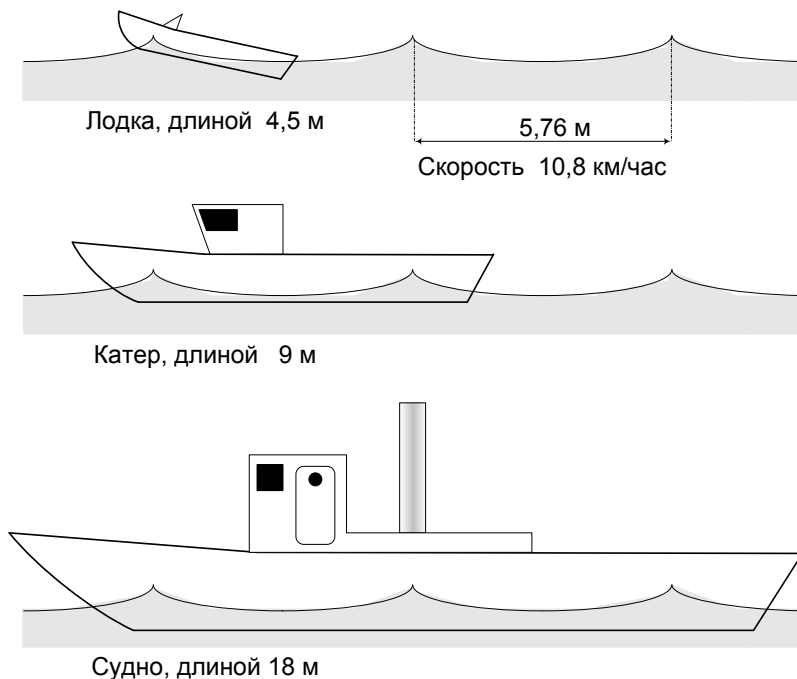
Рисунок 20. «Длина бежит». Чем длинней ватерлиния судна, тем меньше требуется удельная мощность - мощность на единицу водоизмещения
