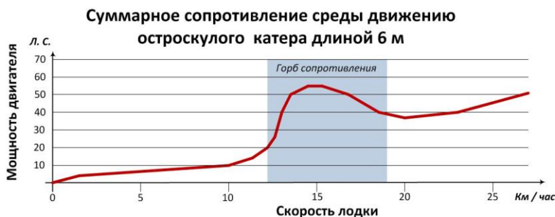
Рисунок 16. Горб сопротивления. Серым цветом отмечена область переходного режима
