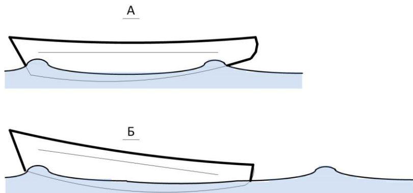
Рисунок 13. Взаимодействие корпуса лодки со своей носовой волновой системой на разных скоростях
